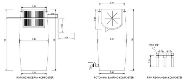
Gambar 3. Potongan depan, samping dan pipa penyangga saringan
