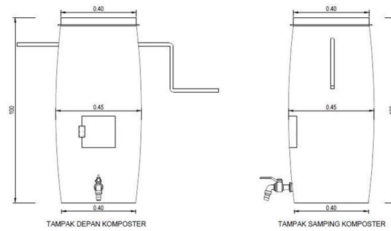
Gambar 2. Tampak depan dan samping komposter
