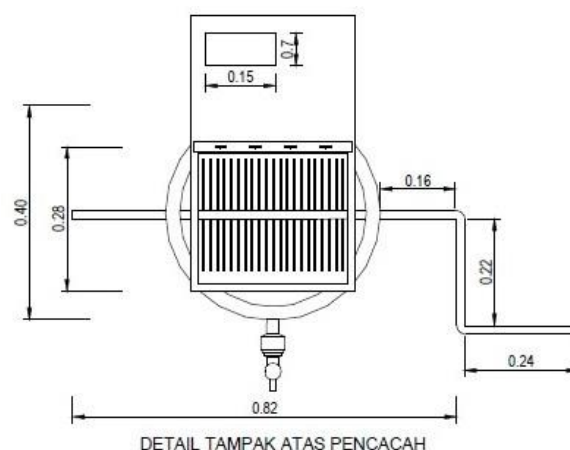
Gambar 1. Detail tampak atas pencacah
