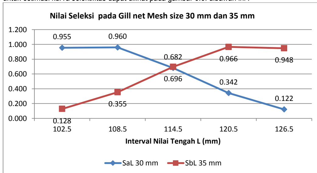
Gambar 3.1. Kurva Seleksi Jaring Insang Hanyut Untuk Ikan Nilem ( Osteocilus hasselti ) di Desa Sungai Batang
